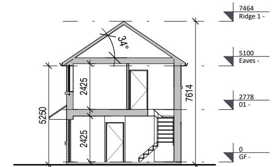
⑦ Section A-A 1 : 200
